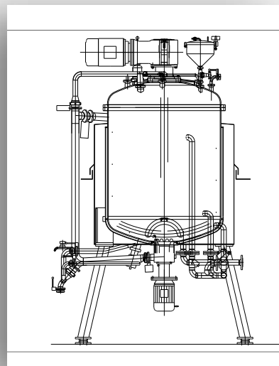
EKATO UNIMIX SRA
